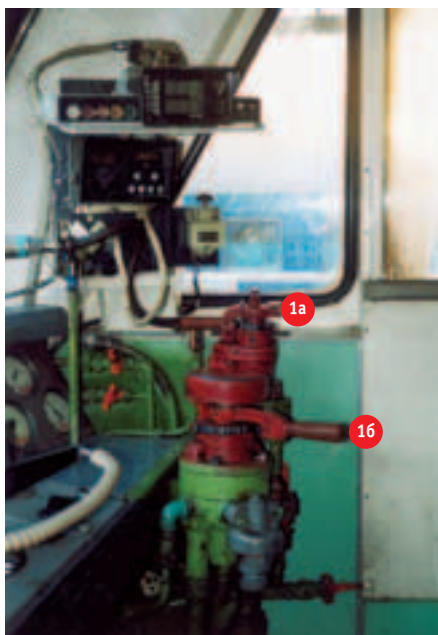
1-а и 1-б: Рычаги тормозов (экстренного и обычного) 2: Штурвал контроля машиниста 3: Датчик контроля внимания машиниста 4: Датчики состояния пневматики
